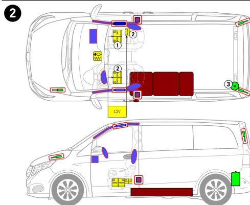
② 附加蓄电池
