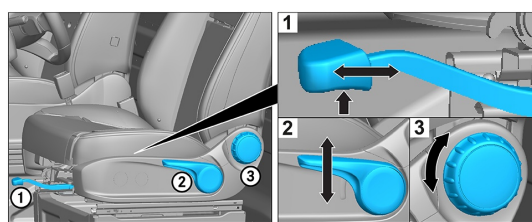
Stolsinställning (mekanisk)
