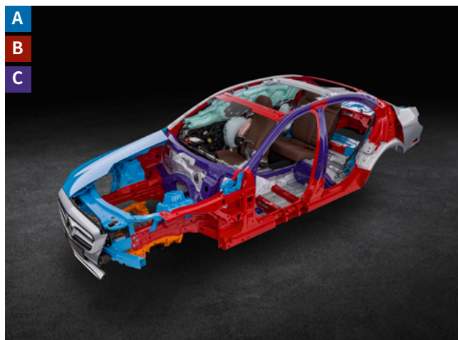
E 级轿车 (213 型) 材料概览示例
