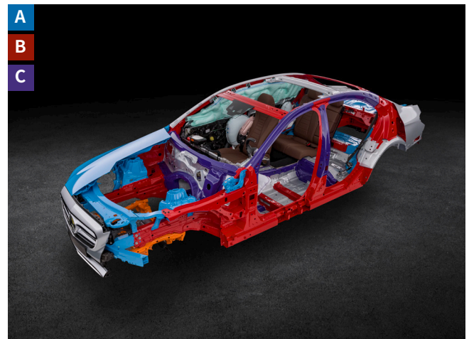
E-클래스 세단(유형 213)의 예를 사용하는 재료 개요
