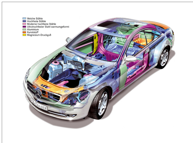
E-클래스 세단(유형 212)의 예를 사용하는 재료 개요
