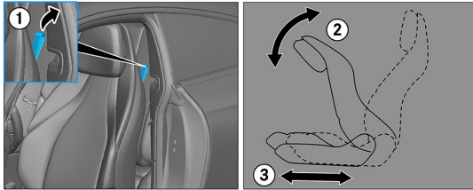
Encosto rebatível do banco dianteiro
