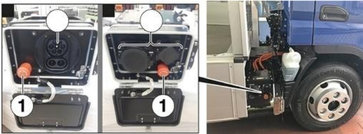
1 NOT-AUS-Taster
