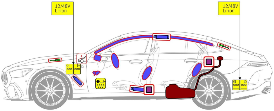
① 12 V/48 V 電池 左駕車輛 ② 12 V/48 V 電池 右駕車輛
