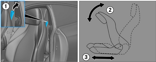
折りたたみ式フロントシートバックレスト
