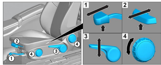
Ülésbeállítás (mechanikus)
