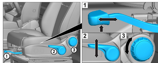
Sitzeinstellung (mechanisch)
