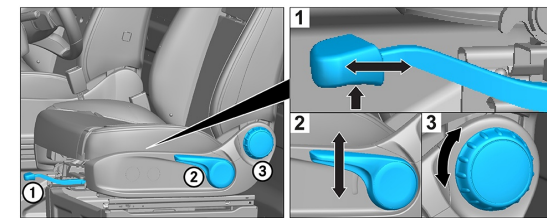
Sitzeinstellung (mechanisch)
