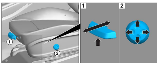
S deindstilling (elektrisk)
